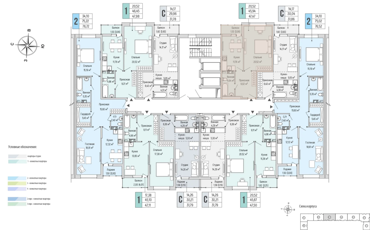
КОРПУС 2. ЭТАЖ 2-9. Планировочные решения. Секция 5.
