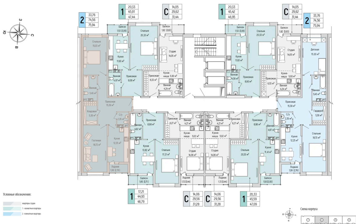
Корпус 3. этаж 3-9. Планировочные решения. Секция 2.
