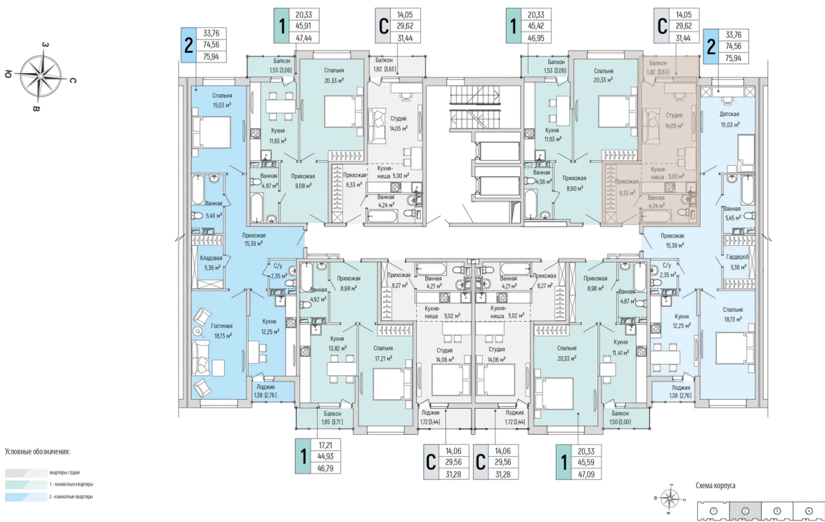
Корпус 3. этаж 3-9. Планировочные решения. Секция 2.
